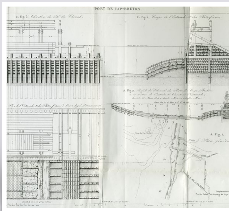
Plan de la construction de l'Estacade par Charles Descombes.
